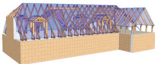
Tagkonstruktion med træspær
